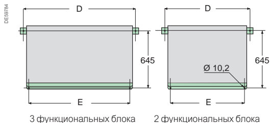
3 функциональных блока
