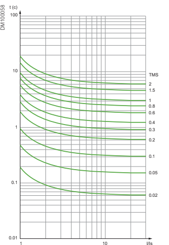
Кривая RI
