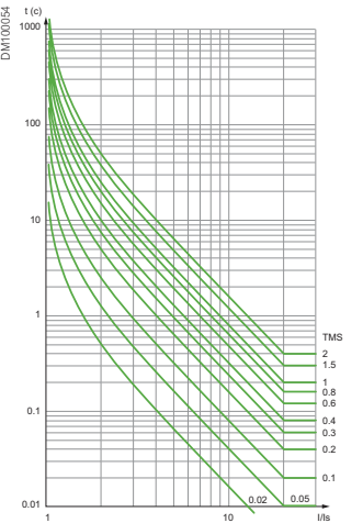
Кривая чрезвычайно обратно-зависимой выдержки времени МЭК (МЭК/EIT или МЭК/C)
