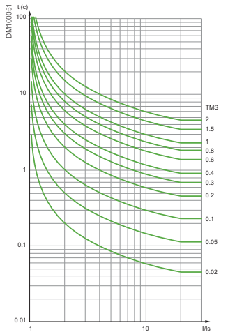
Кривая стандартной обратно-зависимой выдержки времени МЭК (МЭК/SIT или МЭК/A)
