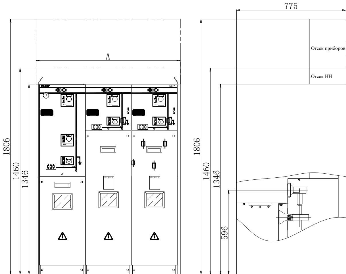
Рис. 2 Габартный чертеж
