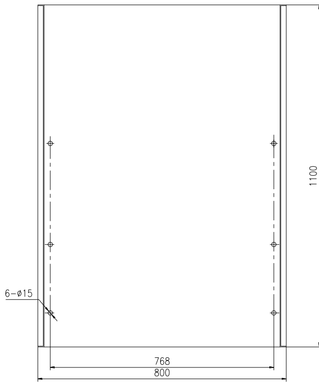
Рис. 9 Габаритный чертеж фундамента ячейки М 12кВ
