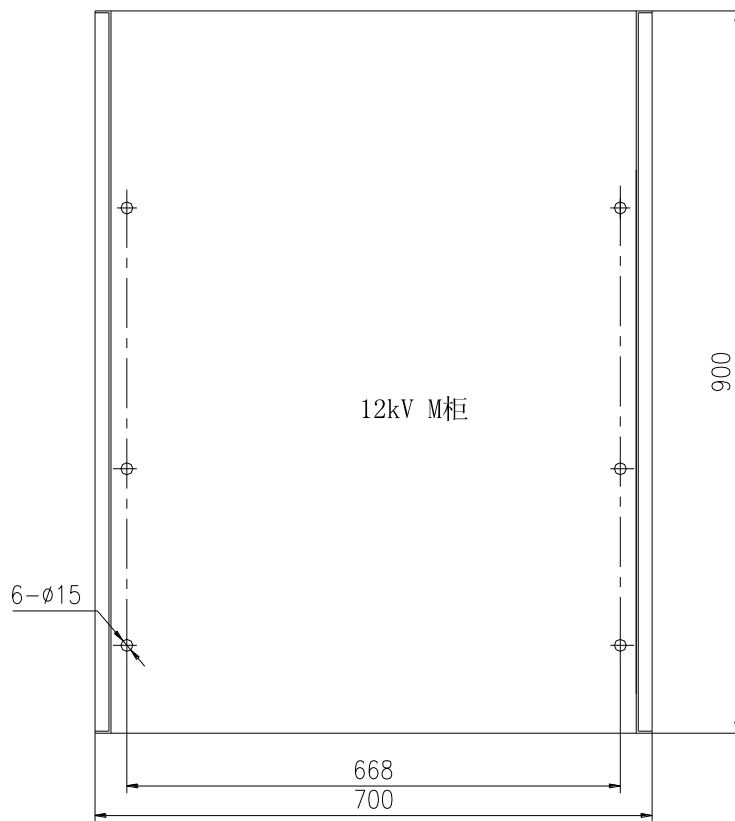
Рис. 10 Габаритный чертеж фундамента ячейки М 24кВ
